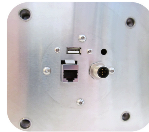
Tragarmsystem (Kabelführung durch Arm)
